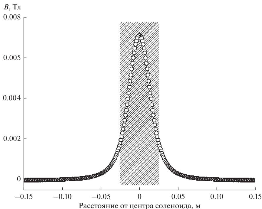
Рис. 3. Зависимость индукции магнитного поля соленооида от расстояния на центральной оси.
