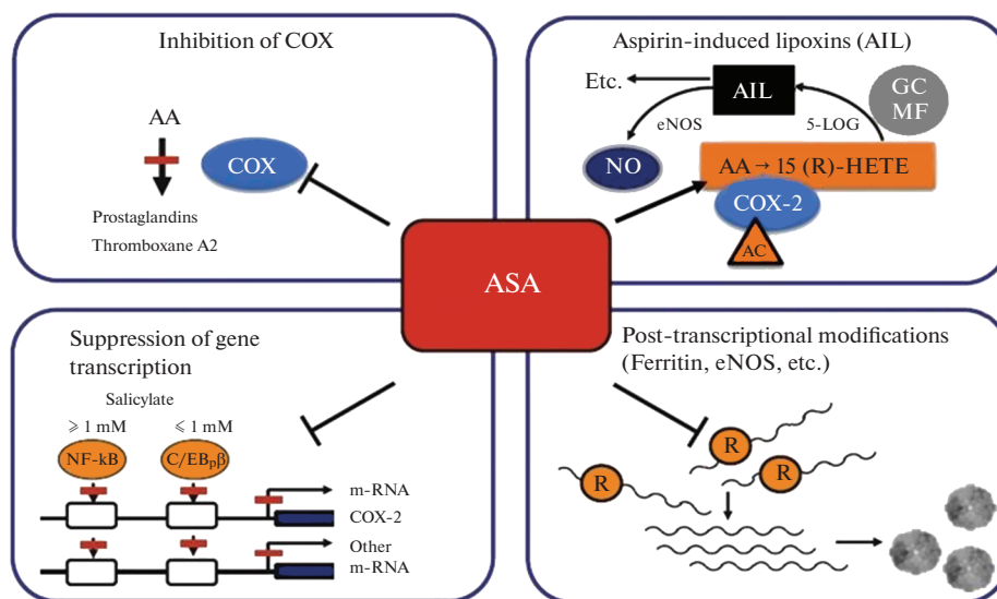
Рис. 1. Механизмы действия аспирина. AA – арахидоновая кислота, ASA – ацетилсалициловая кислота, AC – ацелирование, GC – гранулоциты, MF – макрофаги, COX – циклооксигеназа, AIL – аспирин-индуцированные липоксины, 5-LOG – 5-липоксигеназа, 15-R-HETE – 15-гидрокси-5,8,11,13-эйкозатетраеновая кислота, e-NOS – эндотелиальная синтаза оксида азота, NF-κB – транскрипционный фактор, C/EBPβ – CCAAT-энхансер-связывающий белок, m-RNA – м-РНК (по [49] с модификациями).
