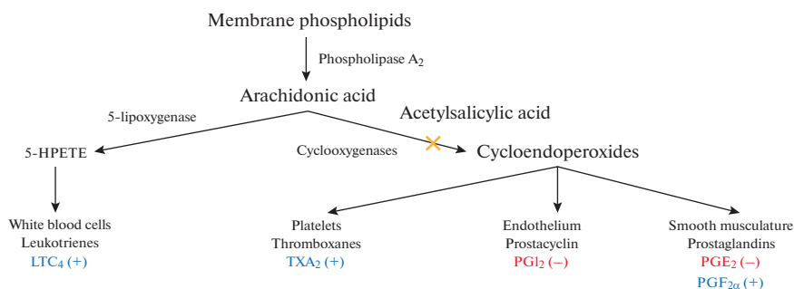
Рис. 2. Схема метаболизма арахидоновой кислоты (+) – вазоконстрикция; (–) – вазодилатация, PGE 2 – простагландин E 2 , PGF 2α – простагландин F 2α , PGI 2 – простагландин I 2 , TXA 2 – тромбосан A 2 , LTC 4 – лейкотриен C 4 , 5-HPETE – 5-гидропероксиэйкозатетраеновая кислота (по [50] с модификациями).
