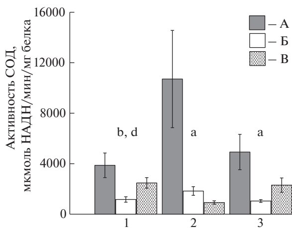
Рис. 2. Активность СОД в тканях сердцевики Cerastoderma glaucum , анадары Anadara kagoshimensis , мидии Mytilus galloprovincialis . Обозначения – как на рис. 1.
