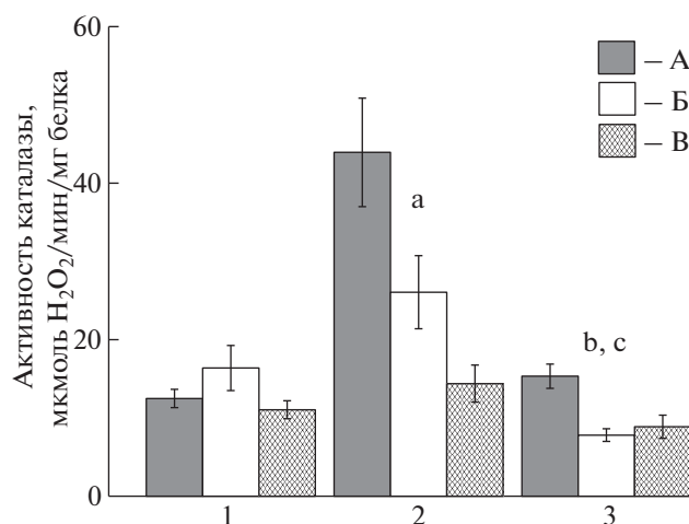
Рис. 3. Активность каталазы в тканях сердцевики Cerastoderma glaucum , анадары Anadara kagoshimensis , мидии Mytilus galloprovincialis . Обозначения – как на рис. 1.
