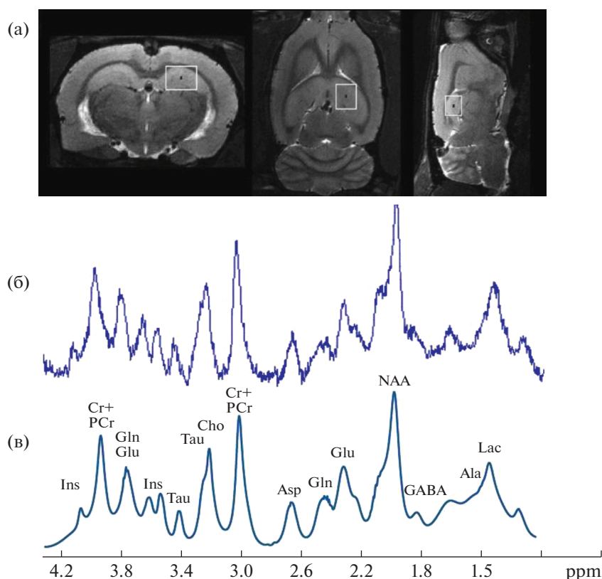
Рис. 2. Расположение области регистрации 1 H спектра нейрометаболитов в головном мозге крыс в трех ортогональных плоскостях (аксональной, сагиттальной и корональной) (а), 1 H спектр до обработки (б), 1 H спектр после обработки (с). Обозначения: Ins – мио-инозитол; Cr – креатинин; PCr – фосфокреатинин; Glu – глутамат; Gln – глутамин; Tau – таурин; Cho – холин-производные; Asp – аспарат; Ala – аланин; Lac – лактат; NAA – N-ацетиласпарат; GABA – γ-аминомасляная кислота.
