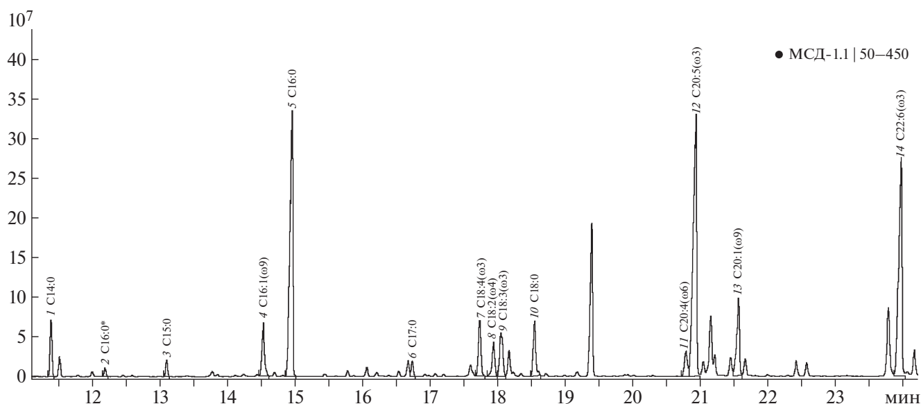
Рис. 1. Хроматограмма МЭЖК, выделенных из сперматозоидов мидии Mytilus galloprovincialis Черного моря. Отмечены кислоты: 1 – миристиновая (C14:0), 2 – 4,8,12-триметилтридекановая, 3 – пентадециловая (C15:0), 4 – пальмитолеиновая (C16:1 \omega 9), 5 – пальмитиновая (C16:0), 6 – маргариновая (C17:0), 7 – стеариноновая (C18:4 \omega 3), 8 – 11,14-октадекадиеновая (C18:2 \omega 4), 9 – \alpha -линоленовая (C18:3 \omega 3), 10 – стеариновая (C18:0), 11 – арахидоновая (C20:4 \omega 6), 12 – эйкозапентаеновая (C20:5 \omega 3), 13 – гондоевая (C20:1 \omega 9), 14 – цервоновая (C22:6 \omega 3).
