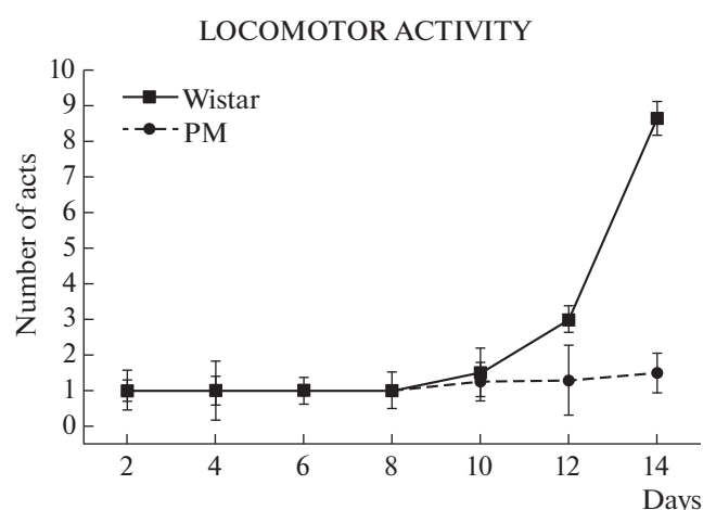
Рис. 3. Локомоторные акты у крыс Вистар и МД. Различия достоверны по влиянию фактора генотипа: F_{(5,237)} = 25.45 ; p < 0.001 .
